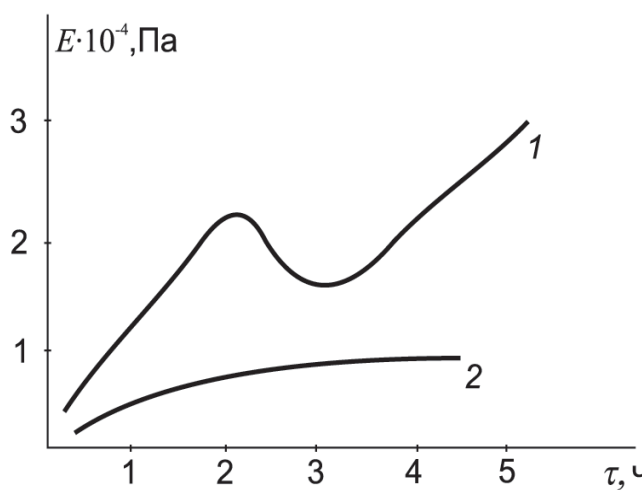
Рис. 1. Кривые изменения во времени \tau модуля быстрой эластической деформации E суспензии MgO: 1 – без поверхностно-активного вещества; 2 – с 1% содержанием лимонной кислоты
