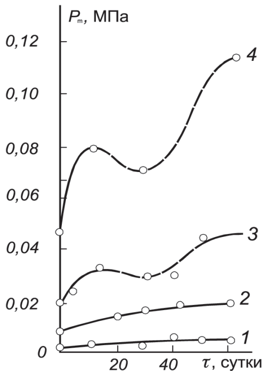
Рис. 3. Зависимость кинетики упрочнения гелей гидросиликатов кальция при C/S = 1,28 от отношения В/Т : 35,18 (1), 19,0 (2), 12,0 (3), 8,7 (4)
